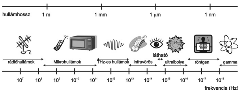
1. ábra * Az elektromágneses spektrum
