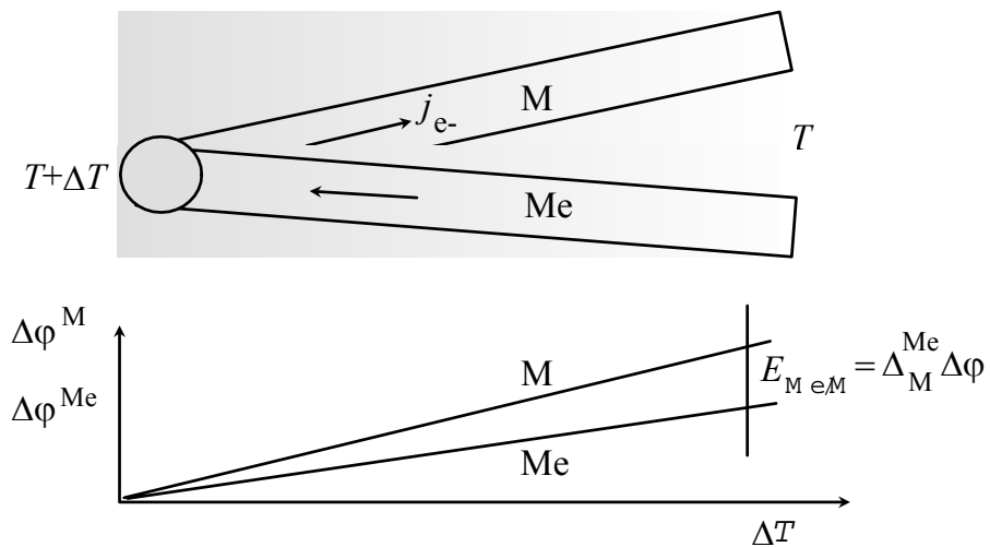
9. ábra: A termofeszültség értelmezése
