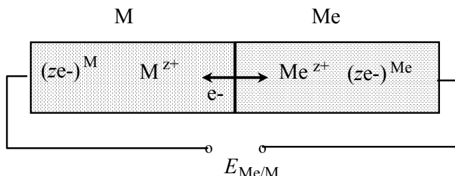
7. ábra: A kontaktpotenciál értelmezése fém-fém között
