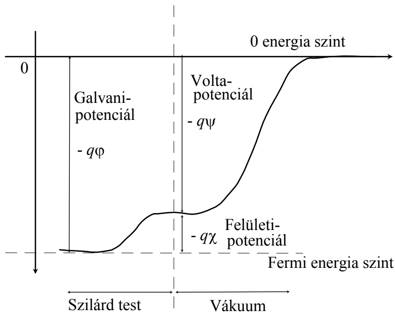
ábra: Az elektron potenciális energiájának változása a fém felületének közelében
