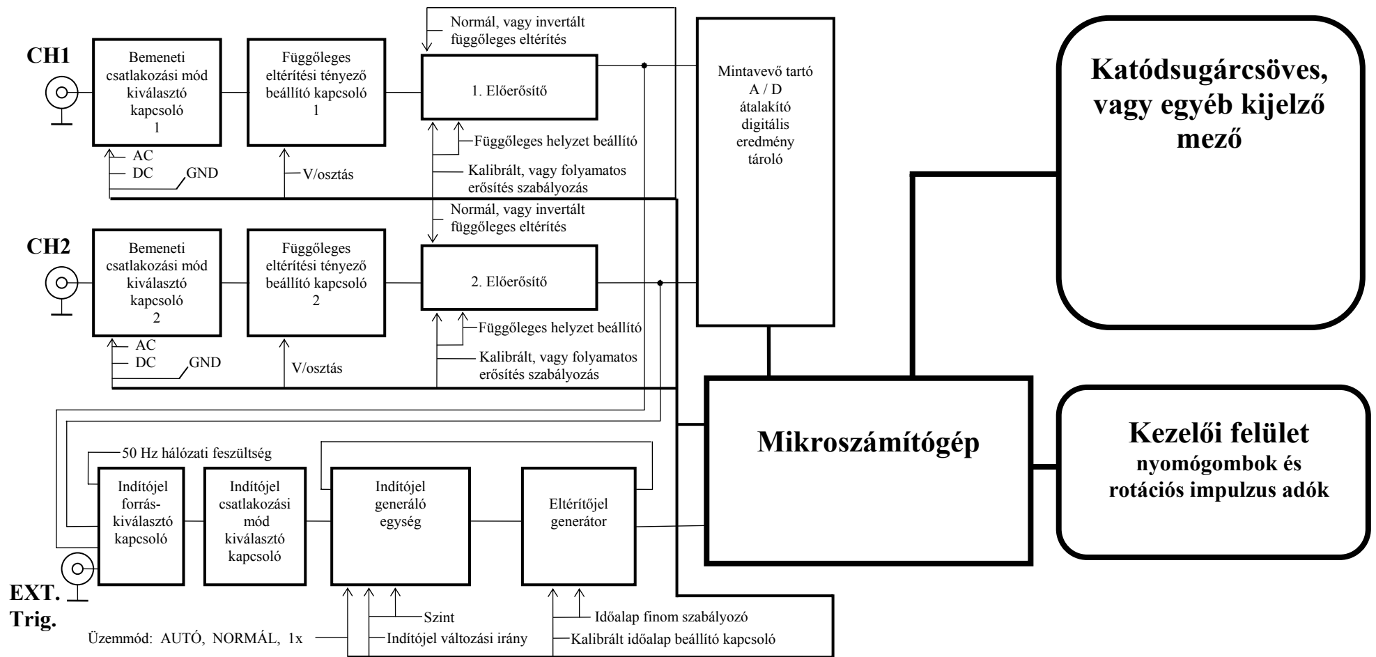
Mai digitális tárolású oszcilloszkóp hatásvázlata. A bemeneti egységeket is mikroszámítógép vezérli.
