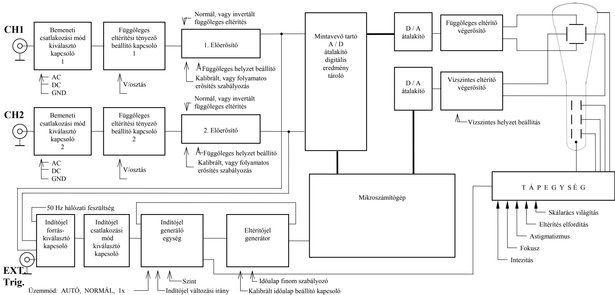
Elektrosztatikus eltérítésű katódsugárcsővel kialakított digitális tárolású oszcilloszkóp hatásvázlata, átmeneti megoldás.
